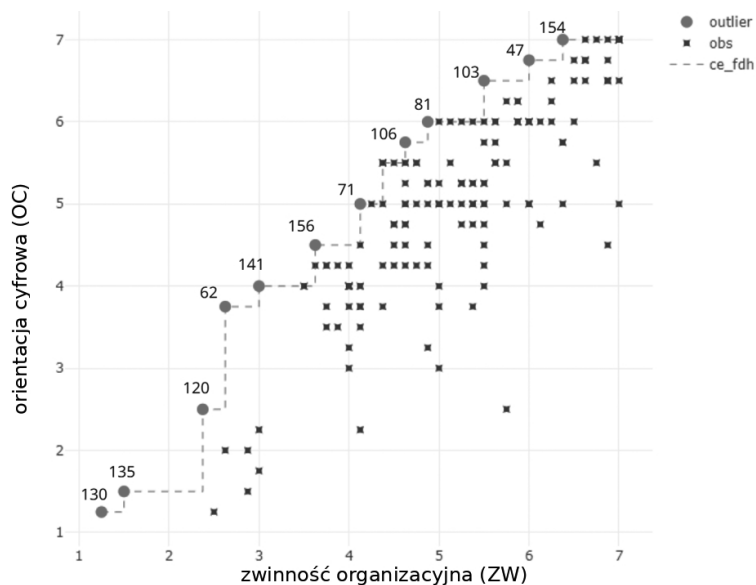
Wykres 12. Wykres potencjalnych obserwacji odstających: zwinność organizacyjna (ZW) – orientacja cyfrowa (OC) ( Y_1 )
