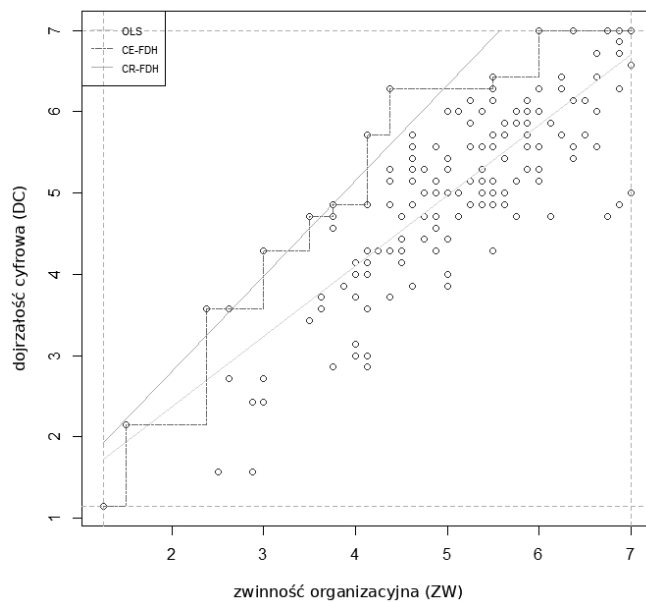
Wykres 8. Wykres NCA: zwinność organizacyjna (ZW) – dojrzałość cyfrowa (DC) ( Y_2 )
