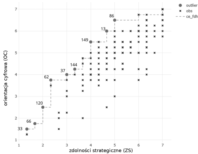
Wykres 13. Wykres potencjalnych obserwacji odstających: zdolności strategiczne (ZS) – orientacja cyfrowa (OC) ( Y_1 )
