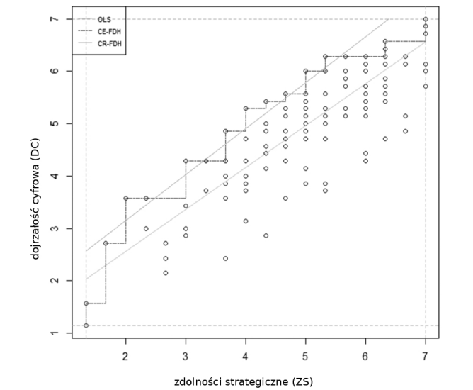
Wykres 9. Wykres NCA: zdolności strategiczne (ZS) – dojrzałość cyfrowa (DC) ( Y_2 )
