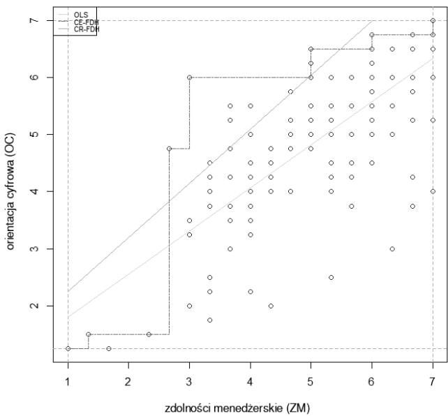
Wykres 6. Wykres NCA: zdolności menedżerskie (ZM) – orientacja cyfrowa (OC) ( Y_1 )
