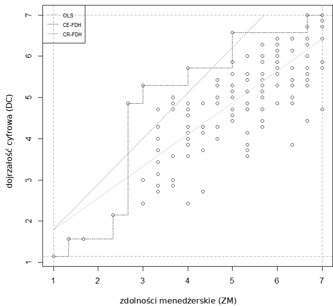
Wykres 10. Wykres NCA: zdolności menedżerskie (ZM) – dojrzałość cyfrowa (DC) ( Y_2 )
