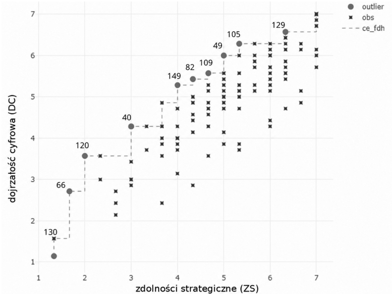
Wykres 17. Wykres potencjalnych obserwacji odstających: zdolności strategiczne (ZS) – dojrzałość cyfrowa (DC) ( Y_2 )
