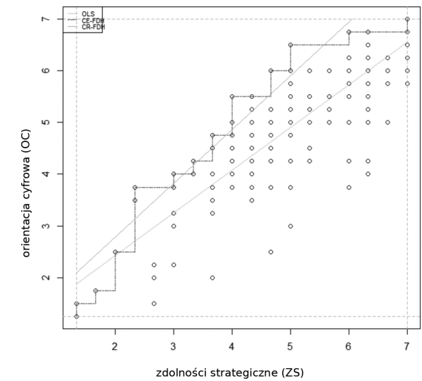
Wykres 5. Wykres NCA: zdolności strategiczne (ZS) – orientacja cyfrowa (OC) ( Y_1 )
