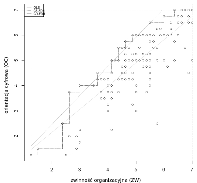
Wykres 4. Wykres NCA: zwinność organizacyjna (ZW) – orientacja cyfrowa (OC) ( Y_1 )
