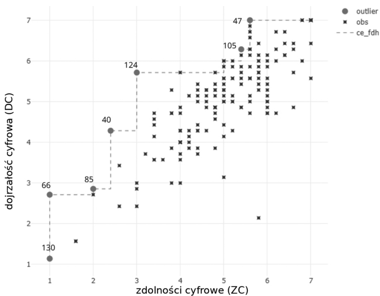
Wykres 15. Wykres potencjalnych obserwacji odstających: zdolności cyfrowe (ZC) – dojrzałość cyfrowa (DC) ( Y_2 )
