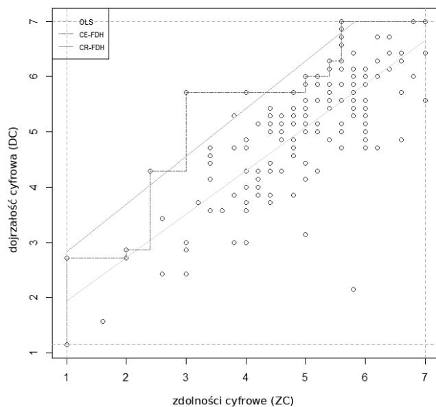
Wykres 7. Wykres NCA: zdolności cyfrowe (ZC) – dojrzałość cyfrowa (DC) ( Y_2 )
