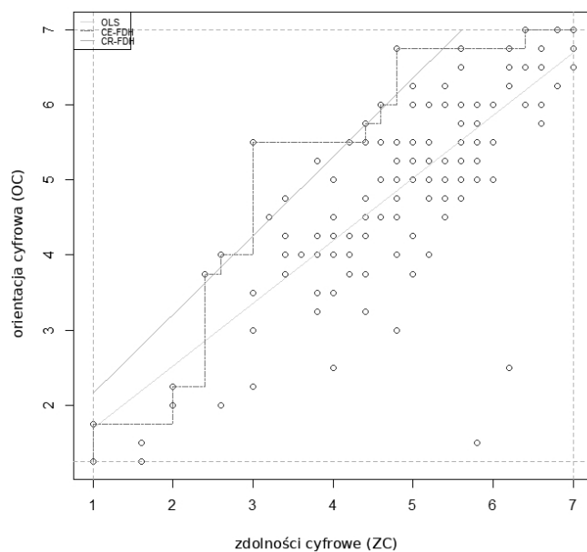
Wykres 3. Wykres NCA: zdolności cyfrowe (ZC) – orientacja cyfrowa (OC) ( Y_1 )
