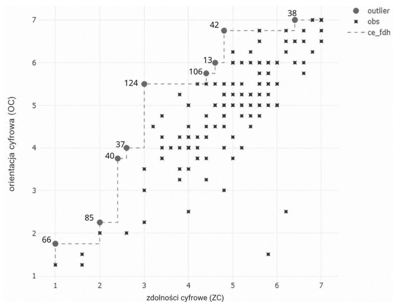
Wykres 11. Wykres potencjalnych obserwacji odstających: zdolności cyfrowe (ZC) – orientacja cyfrowa (OC) ( Y_1 )
