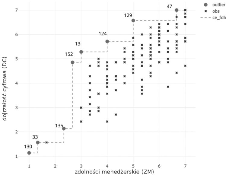
Wykres 18. Wykres potencjalnych obserwacji odstających: zdolności menedżerskie (ZM) – dojrzałość cyfrowa (DC) ( Y_2 )
