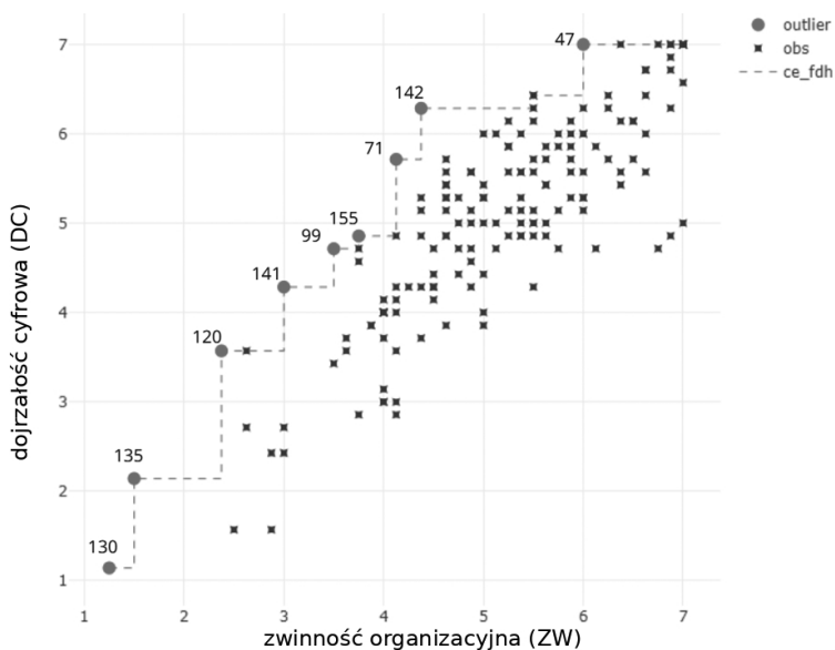
Wykres 16. Wykres potencjalnych obserwacji odstających: zwinność organizacyjna (ZW) – dojrzałość cyfrowa (DC) ( Y_2 )
