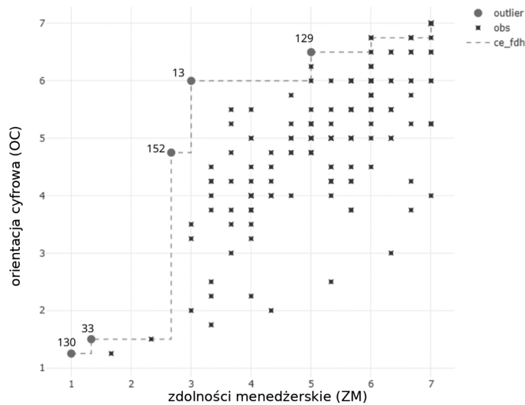
Wykres 14. Wykres potencjalnych obserwacji odstających: zdolności menedżerskie (ZM) – orientacja cyfrowa (OC) ( Y_1 )
